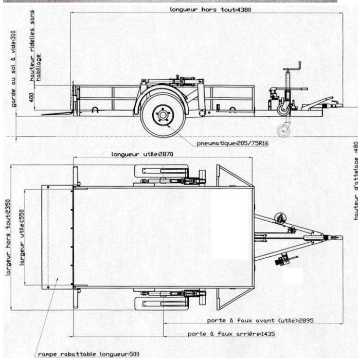
Dimensions de la version standard
